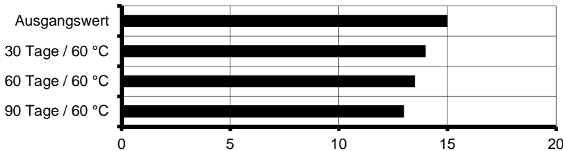
Durchschnittliche Zugscherfestigkeit (N/mm 2 ) - nach Lagerung unter Wärmeeinfluss -
