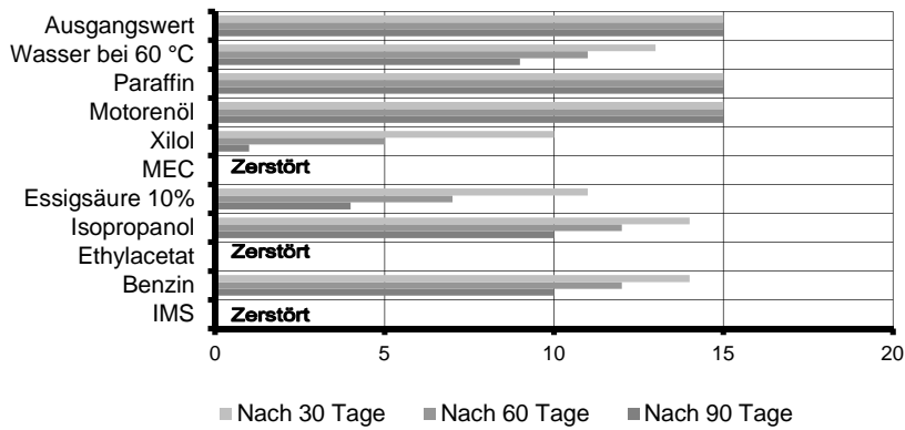
Durchschnittliche Zugscherfestigkeit (N/mm 2 ) - nach Lagerung in diversen Medien -
