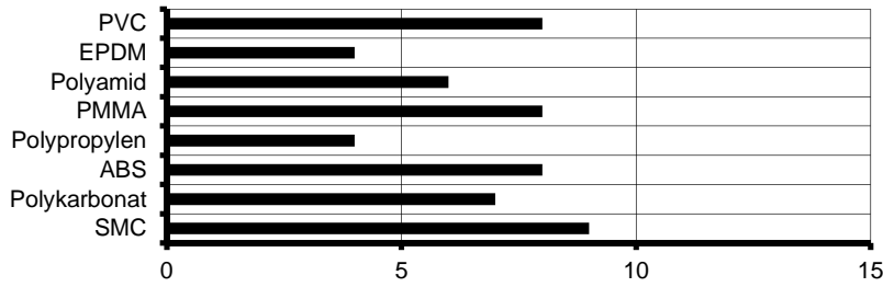
Durchschnittliche Zugscherfestigkeit (N/mm 2 ) - von Kunststoffen -
